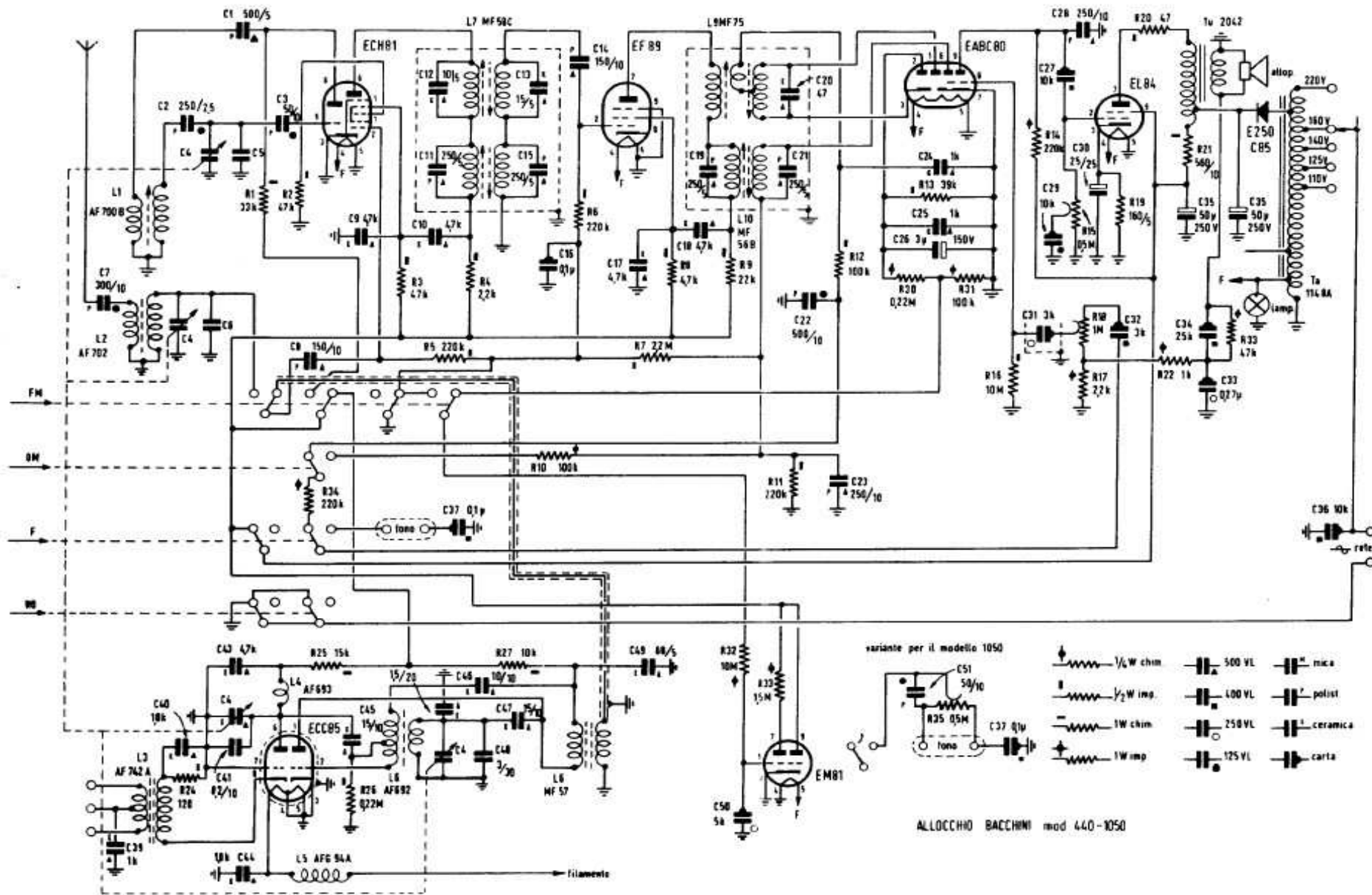
Schema elettrico del radiorecettore ALLOCCHIO BACCHINI, mod. 440 - 1050
